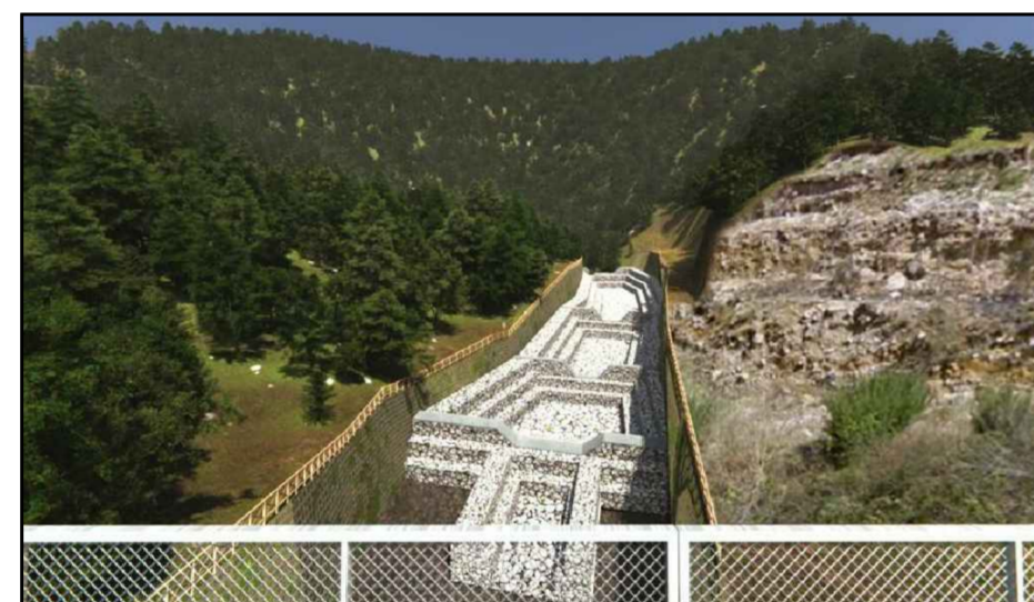
VISTA 3 Vasca 3 - Rendering
